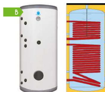
BOILER ECS ÉMAILLÉ LIFE PLUS
