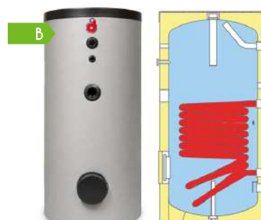
BOILER ECS ÉMAILLÉ LIFE
