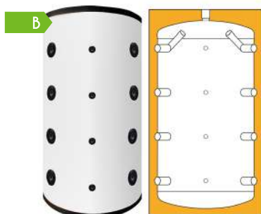
TAMPON DE CHAUFFAGE BUFFER 200L
