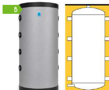
BOUTEILLE DE MÉLANGE MURALE
