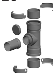
TE 87° D'ETAGE Ø 110 AVEC 1x PIQUAGE Ø80
