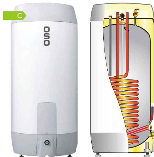
BOILER ÉLECTRIQUE INOX OSO SUPER COIL
