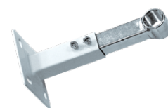
SUPPORT TÉLÉSCOPIQUE POUR VASE JUSQU'À 40L 3/4"
