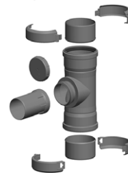
T-STUK 87° VERDIEPING Ø 110 X 1 AFTAKKING Ø 80
