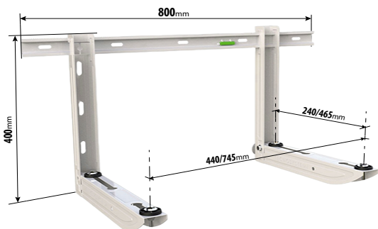
VOORGEMONTEEDE MUURBEUGEL-GALILEO-100KG
